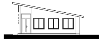
ELEVACIÓN NORTE ESCALA 1:50
