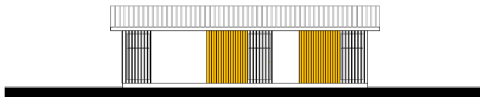
ELEVACIÓN SUR ESCALA 1:50
