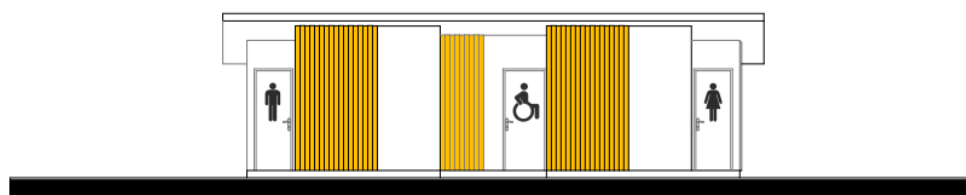
ELEVACIÓN NORTE ESCALA 1:50
