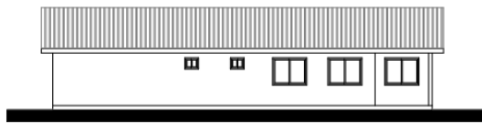
ELEVACIÓN OESTE ESCALA 1:50
